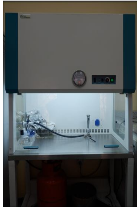
كابينة التعقيم Laminar Flow
